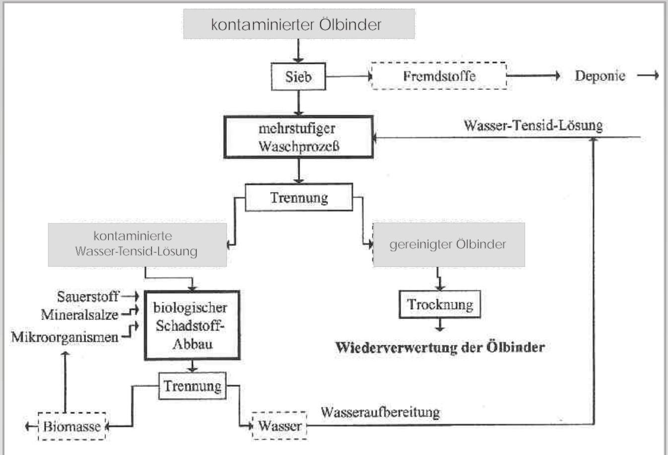
Übersichtsschema für die Behandlung kontaminierter Ölbinder mit dem Ziel von deren Wiederverwertung
